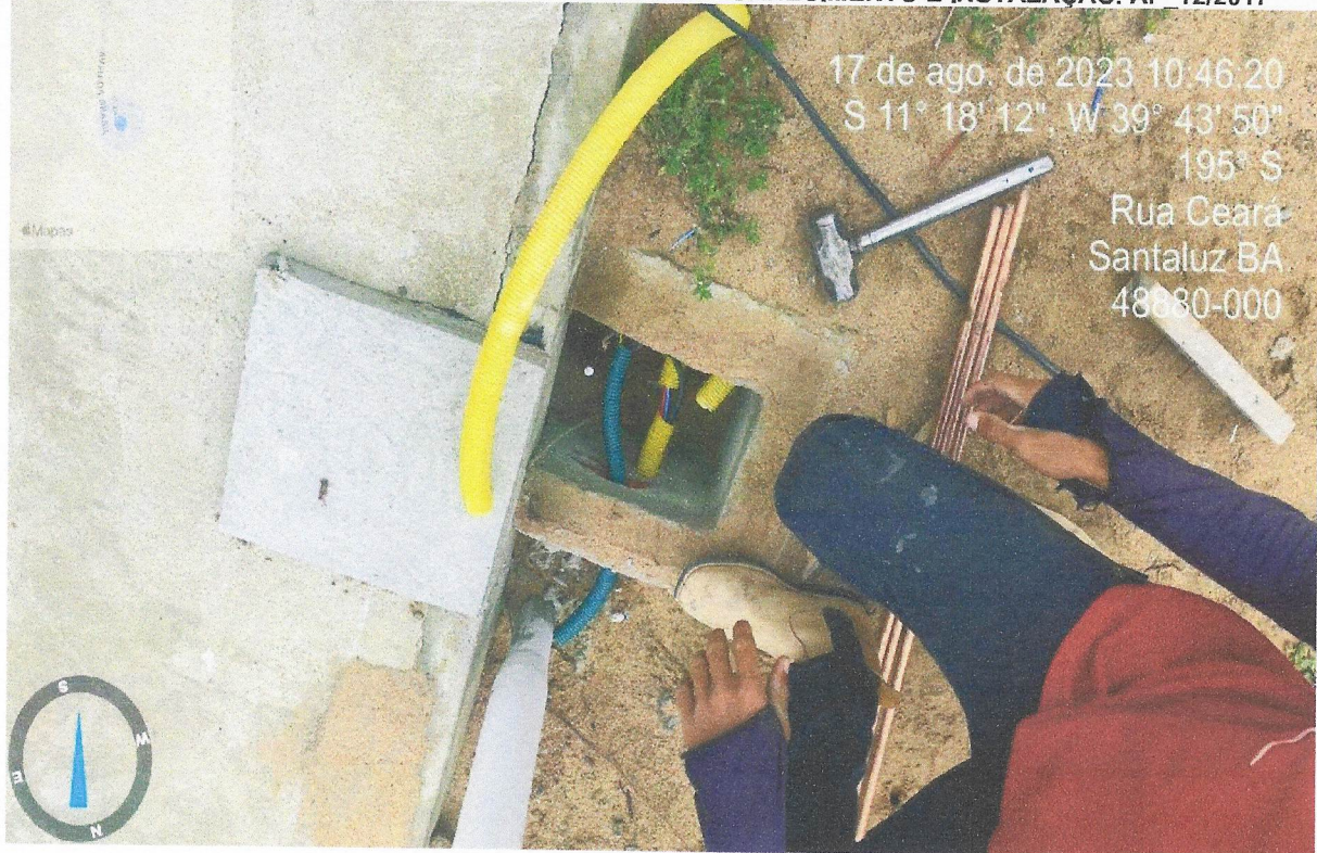
FOTO 12 - "HASTE DE ATERRAMENTO 5/8 PARA SPDA - FORNECIMENTO E INSTALAÇÃO. AF_12/2017"
